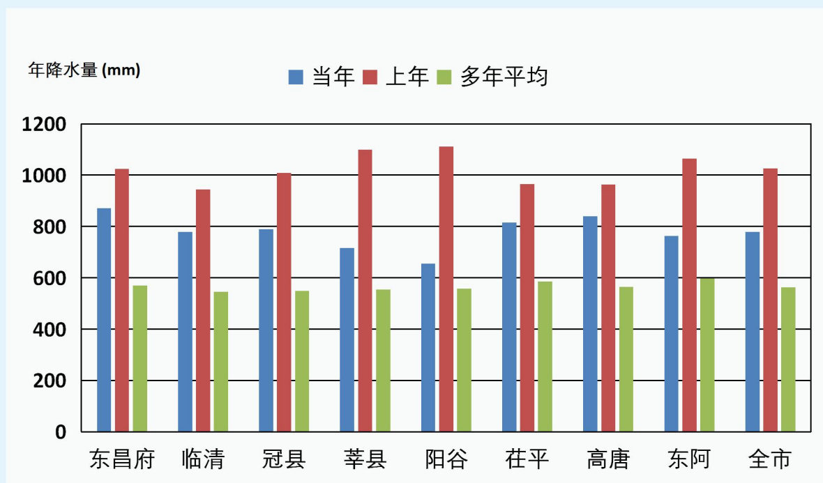
图 1 2022 年聊城市各县（市、区）年降水量与上年及多年平均比较图
