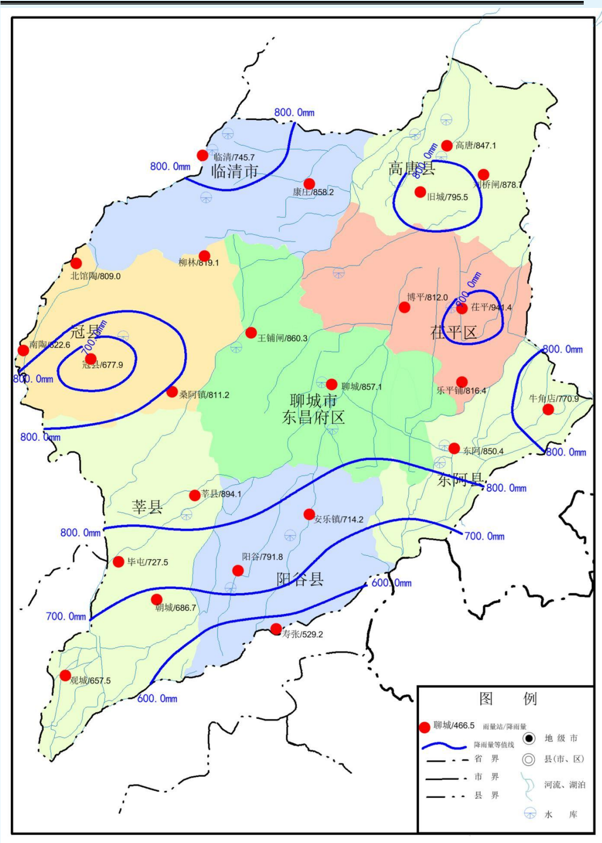
图 2 聊城市 2022 年年降水量等值线图
